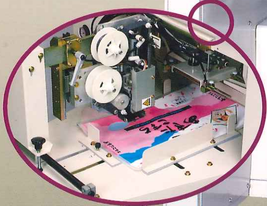
オプション:印字装置
